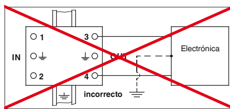
Conexión de tierra
