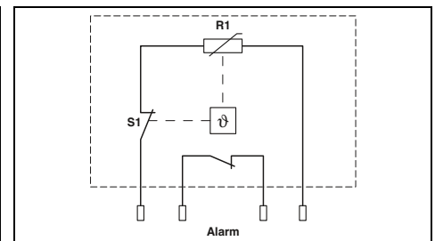
Aplicaciones de 1500 V DC y 690 V AC, con indicación óptica y contacto de indicación remota, aislamiento doble
