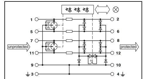
5 conductores con potencial de referencia conjunto, conexión 9/10 con toma a tierra directa
