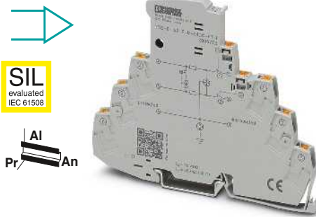
Circuito de dos hilos (loop), sin potencial de tierra, conexión 3/6 mediante descargador de gas puesto a tierra, con interrupción por cuchilla, p. ej. para bucles de corriente de 4 ... 20 mA
