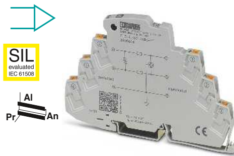
Circuito de dos hilos (loop), sin potencial de tierra, conexión 3/6 con puesta a tierra directa, p. ej. para bucles de corriente de 4 ... 20 mA
