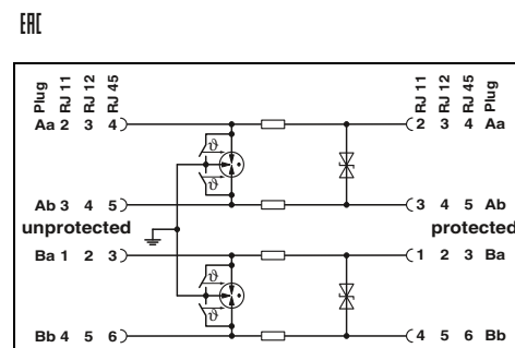
Conector intermedio para dos interfaces SHDSL (puertos)
