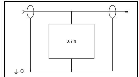
Para instalaciones GSM (0,8 GHz–2,25 GHz), pantalla puesta a tierra, conexión: tipo N
