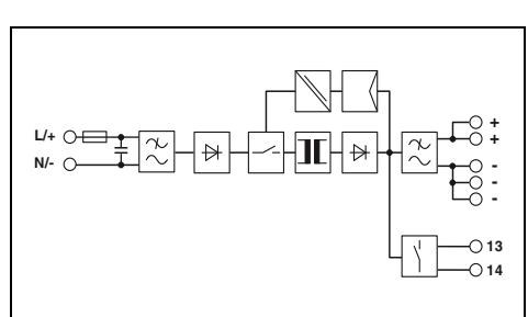
Fuente de alimentación, 1 AC, 24 V DC, 3 A NEC Class 2
