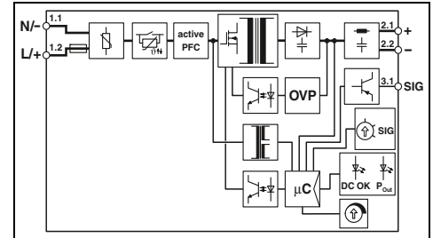
Fuente de alimentación, 1 AC, 24 V DC, 1,3 A, SC NEC clase 2
